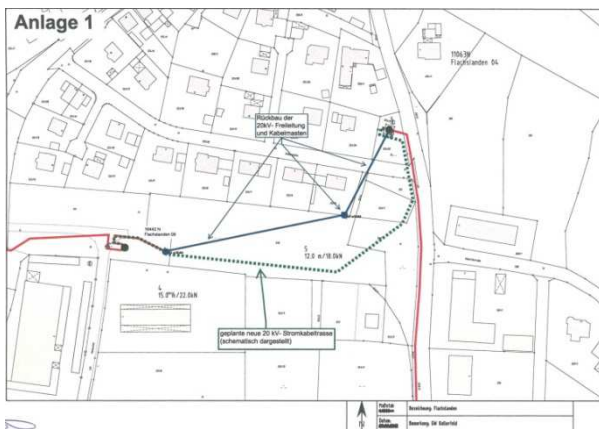
Plan der Verlegung der Freileitung
