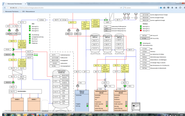
Die Anlagenübersicht über das Wärmenetz Flachslanden
