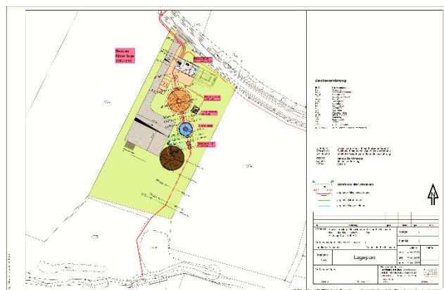
Planung des Neubaus der Kläranlage Flachslanden
