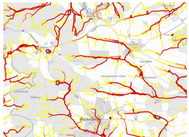
Abbildung 1: Ausschnitt aus dem Umweltatlas (umweltatlas.bayern.de) Themen: Potentielle Fließwege bei Starkregen; Geländesenken und potentielle Aufstaubereiche und Wassersensible Bereiche
